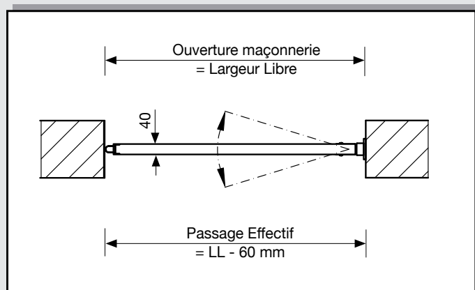
Montage maçonnerie
