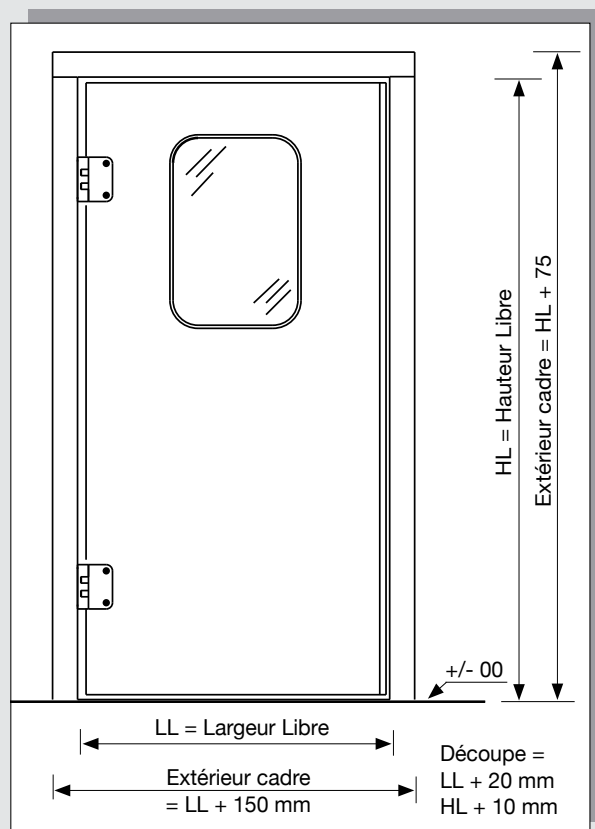
Montage panneaux
