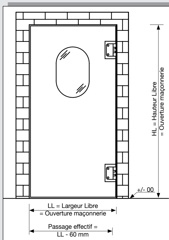
Montage maçonnerie
