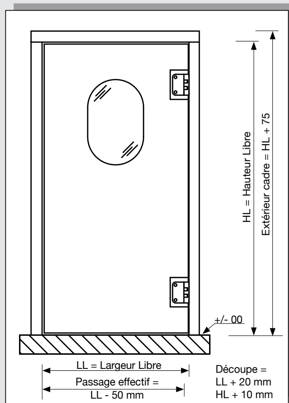
Montage panneaux
